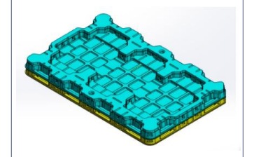
ハーフカット型トレイ 16
