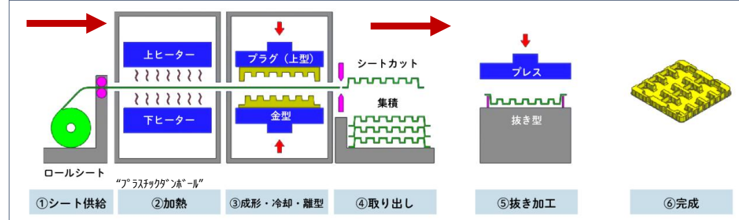
自由設計プラダン 14
