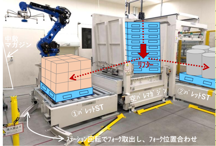
全自動①パレタイズRoboと②パレタイズRobo
